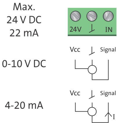
Fig. 41 Wiring, analog input
