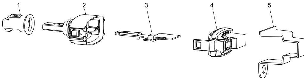
Fig. 34 Sensor
